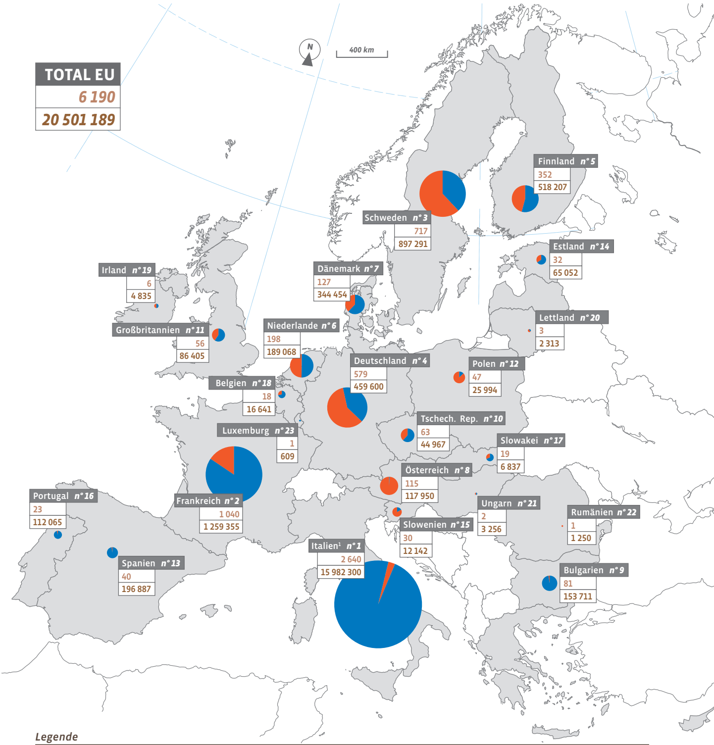
Erneuerbare Energiegewinnung durch Wärmepumpen (in ktoe) und Anzahl in Betrieb befindlicher Wärmepumpen in der Europäischen Union 2012
