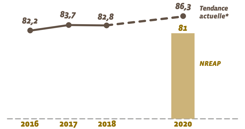
Tendance actuelle de la consommation de chaleur issue de biomasse solide par rapport à la feuille de route des plans d'action nationaux énergies renouvelables (en Mtep)
